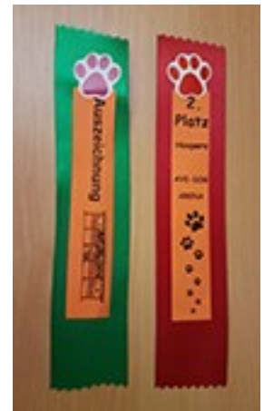
Ausgezeichnet-Schleife + Platzierungs-Schleife
